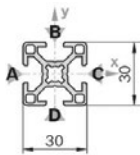
30x30 Strut
