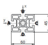
45x60 Strut
