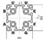
90x90L Strut
