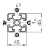
45x45L Strut
