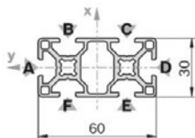
30x60 Strut
