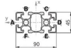
45x90L Strut
